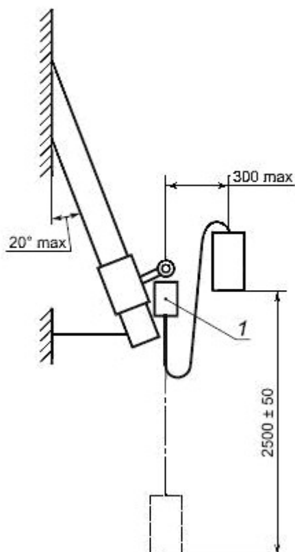
Рисунок 9 - Проверка динамической характеристики анкерных устройств, закрепляемых на наклонных крышах
