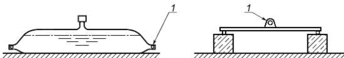
Рисунок 6 - Класс E. Примеры анкерных устройств с противовесом
