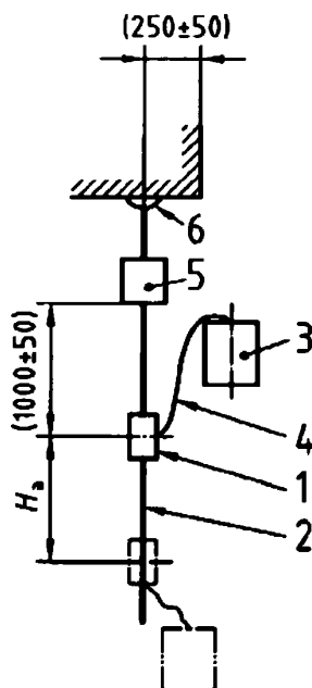
1 — устройство позиционирования на канатах; 2 — анкерный канат; 3 — жесткая стальная масса; 4 — стропа; 5 — устройство измерения силы; 6 — анкерная точка а; H_a — страховочный участок
