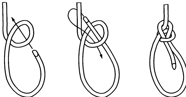
Рисунок 3 — Узел булинь
